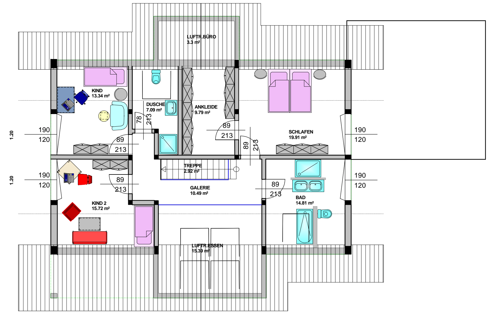
DACHGESCHOSS
