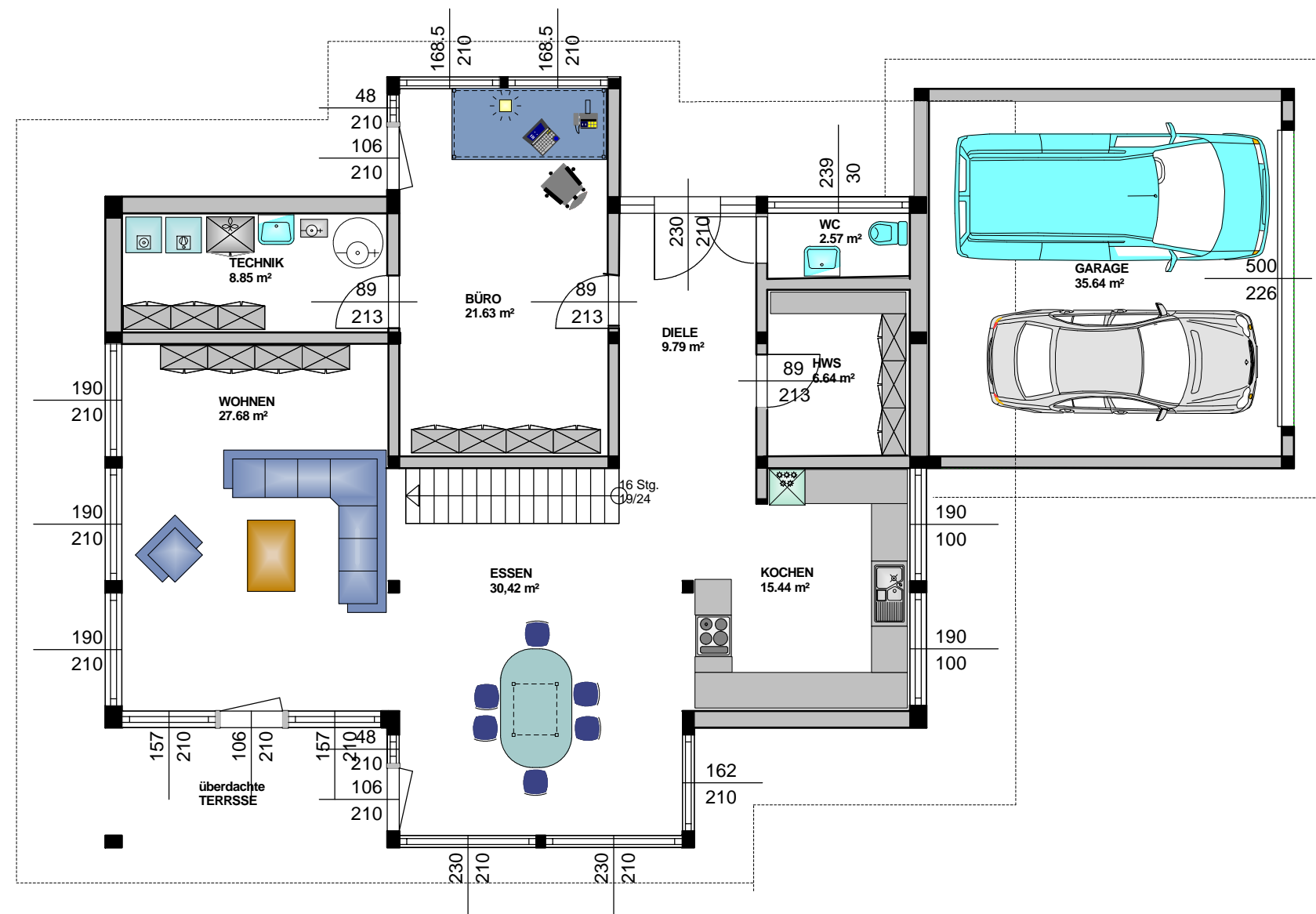
ERDGESCHOSS
