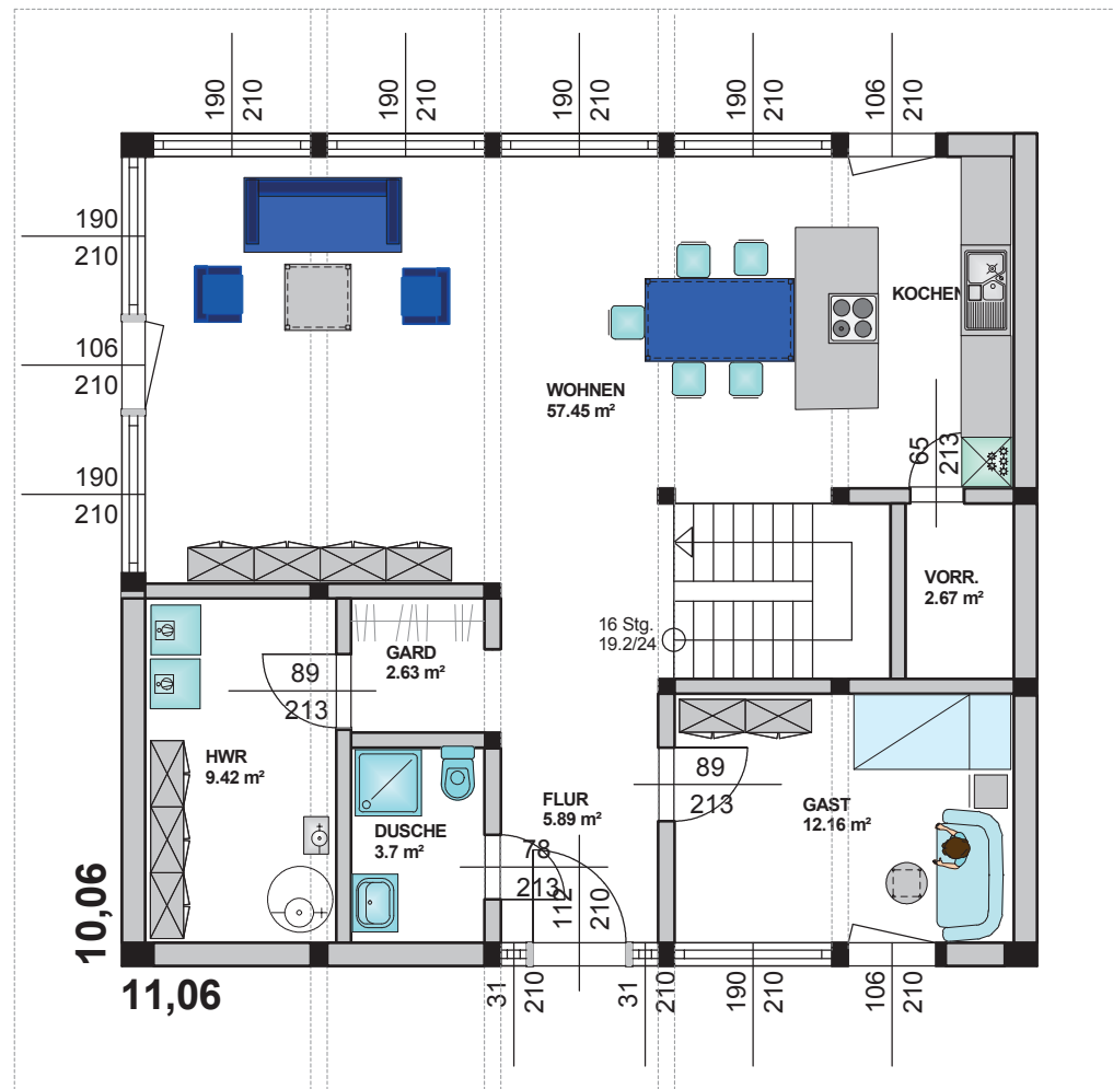
ERDGESCHOSS
