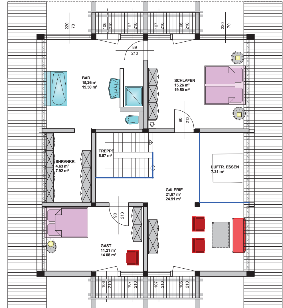
DACHGESCHOSS
