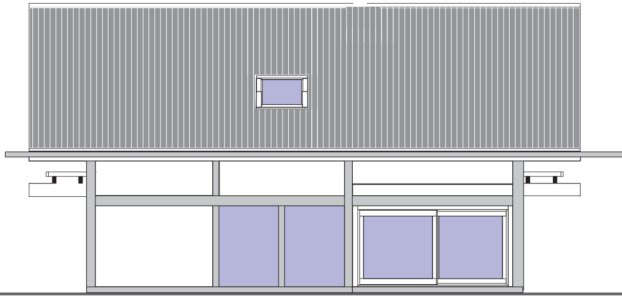
OSTANSICHT
