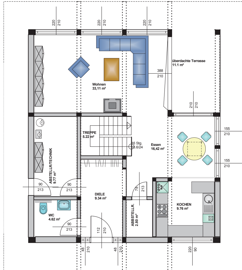
ERDGESCHOSS
