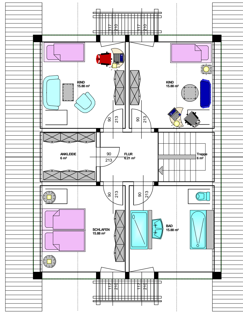
DACHGESCHOSS
