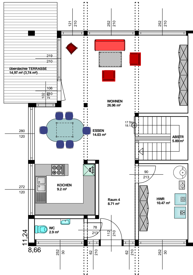
ERDGESCHOSS
