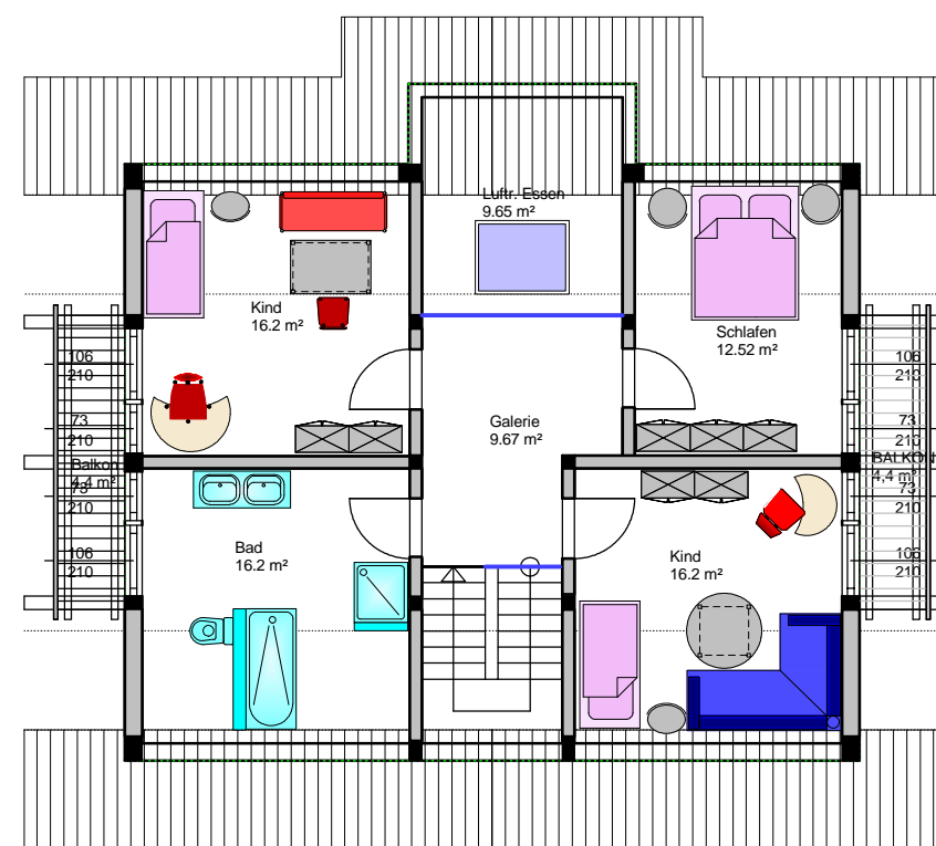
DACHGESCHOSS
