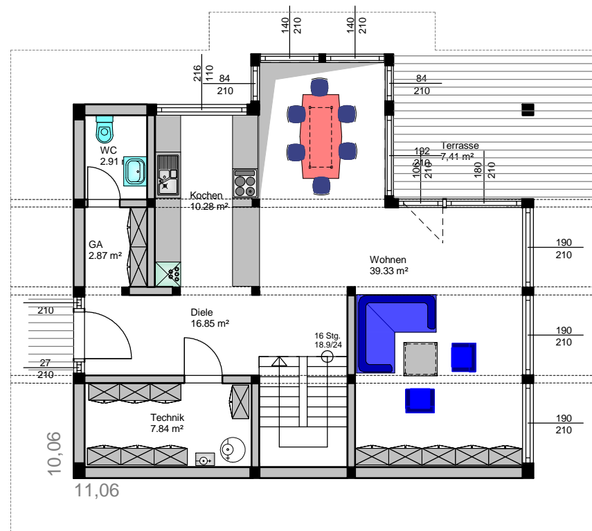
ERDGESCHOSS
