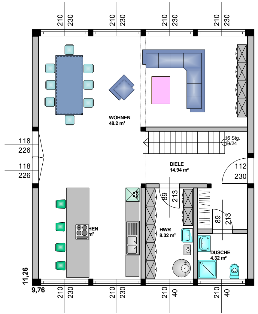
ERDGESCHOSS
