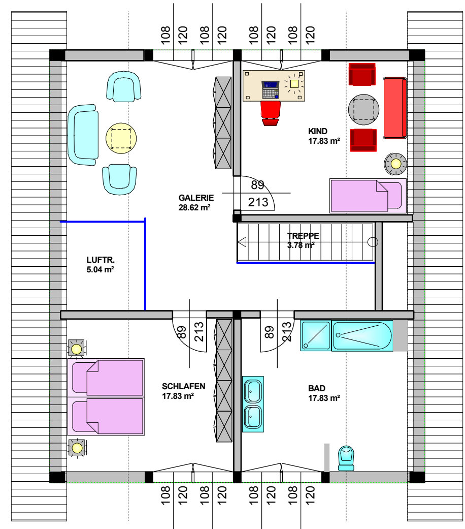
DACHGESCHOSS
