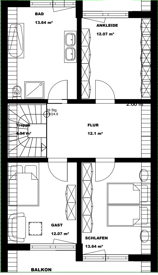
DACHGESCHOSS
