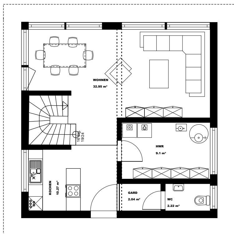
ERDGESCHOSS
