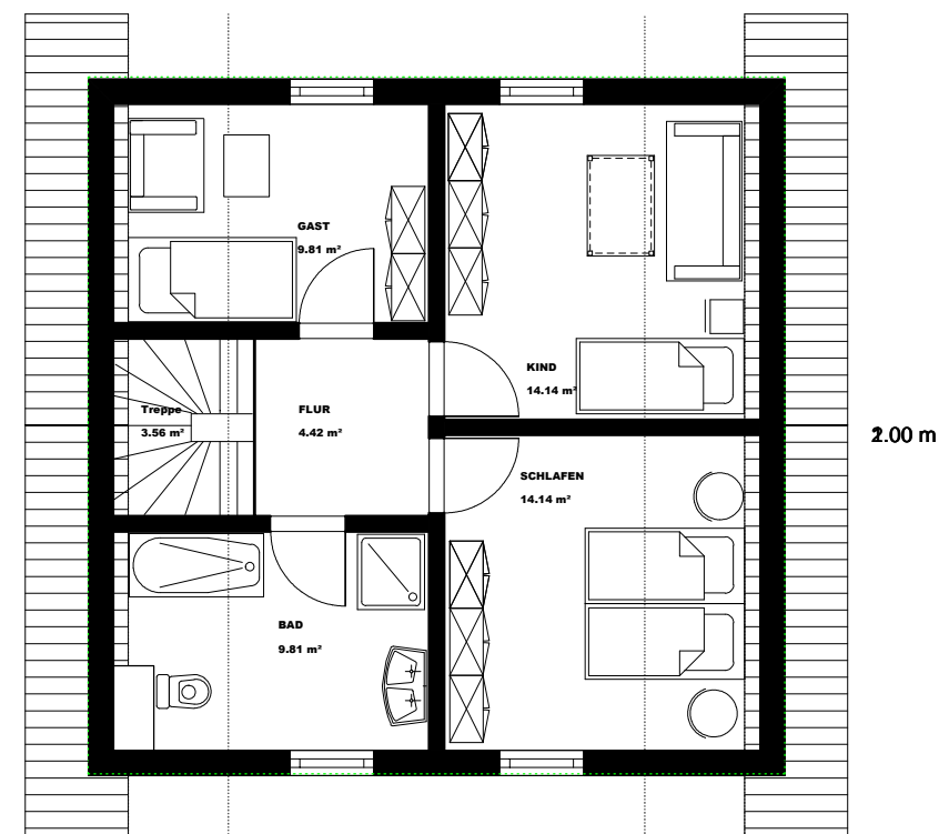
DACHGESCHOSS
