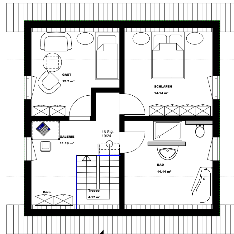
DACHGESCHOSS
