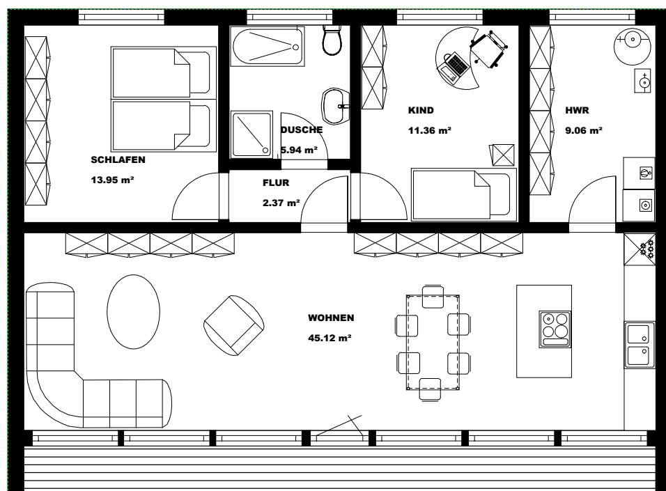
ERDGESCHOSS
