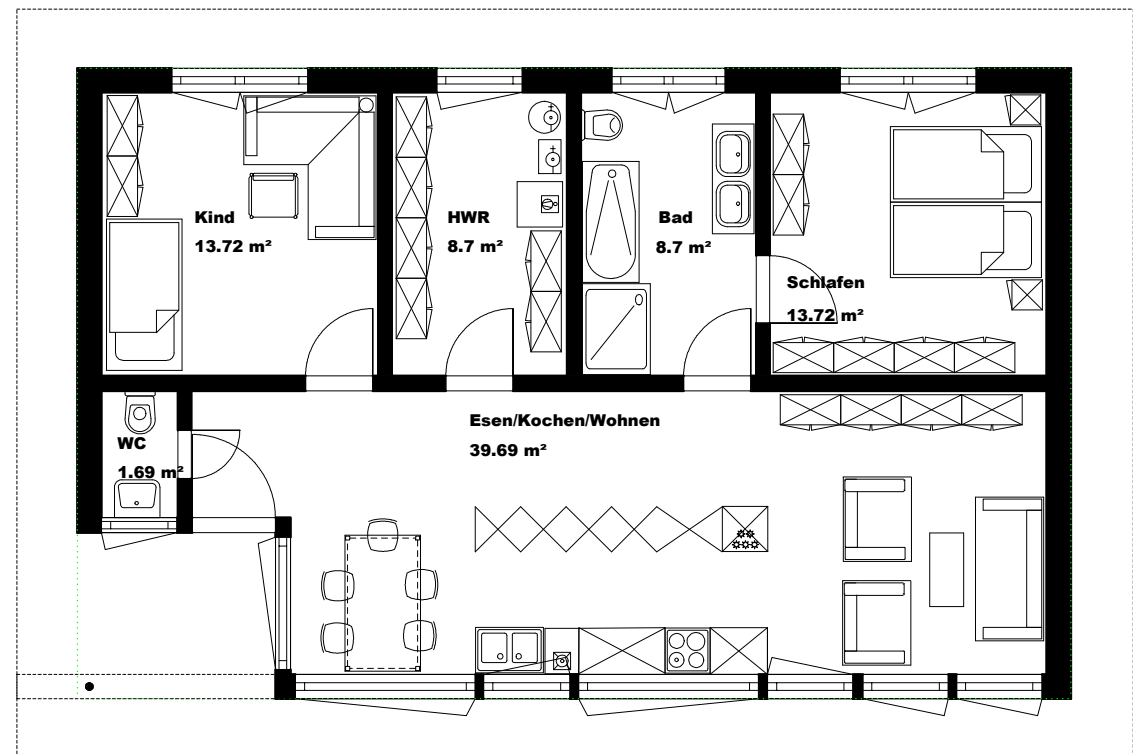
ERDGESCHOSS
