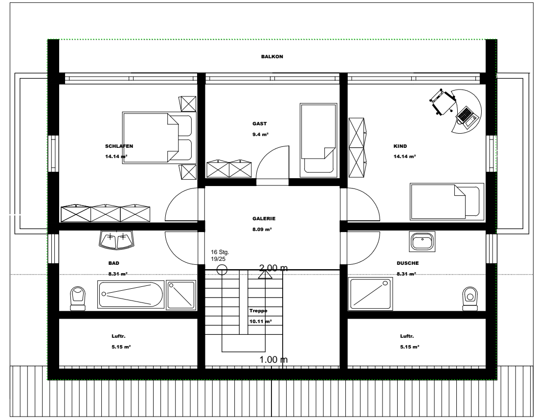
DACHGESCHOSS
