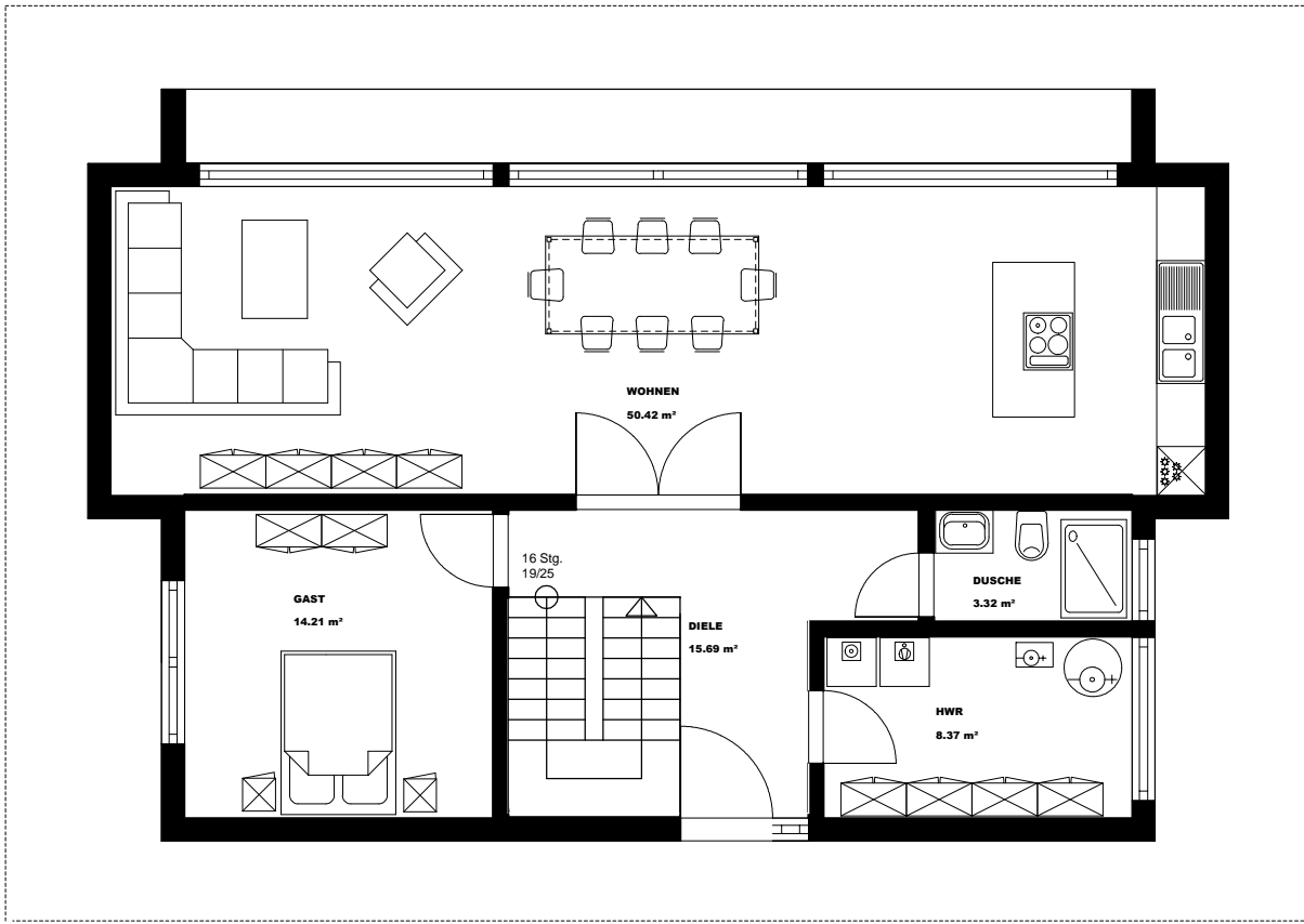
ERDGESCHOSS
