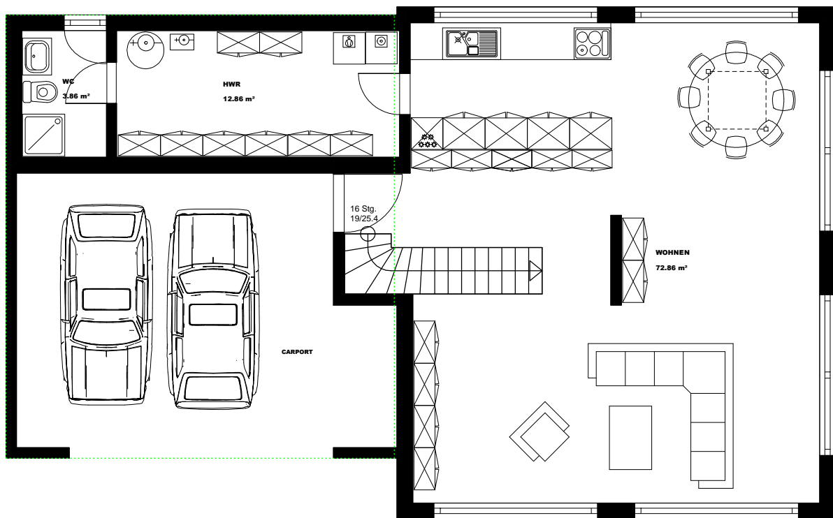
ERDGESCHOSS
