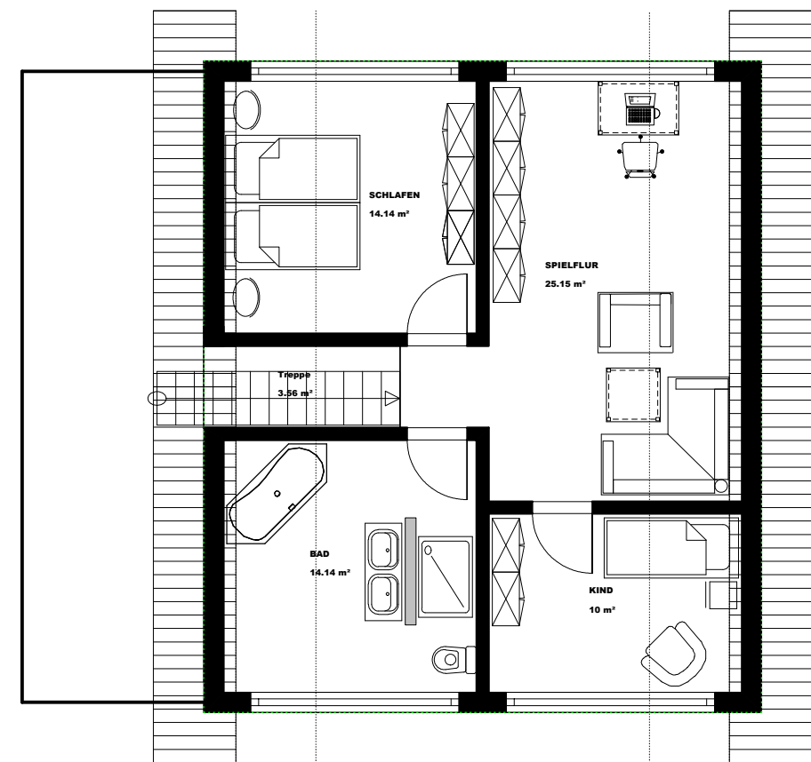
DACHGESCHOSS
