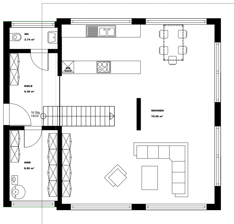
ERDGESCHOSS
