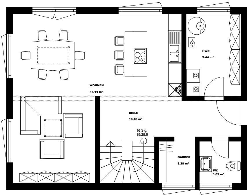
ERDGESCHOSS
