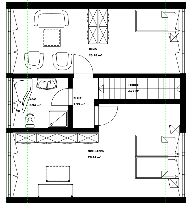
DASCHGESCHOSS
