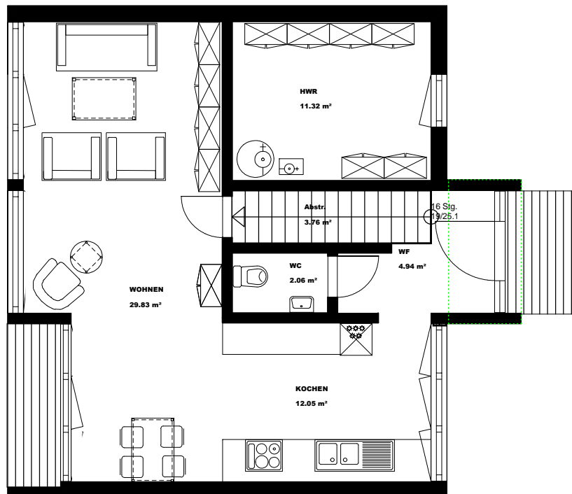
ERDGESCHOSS
