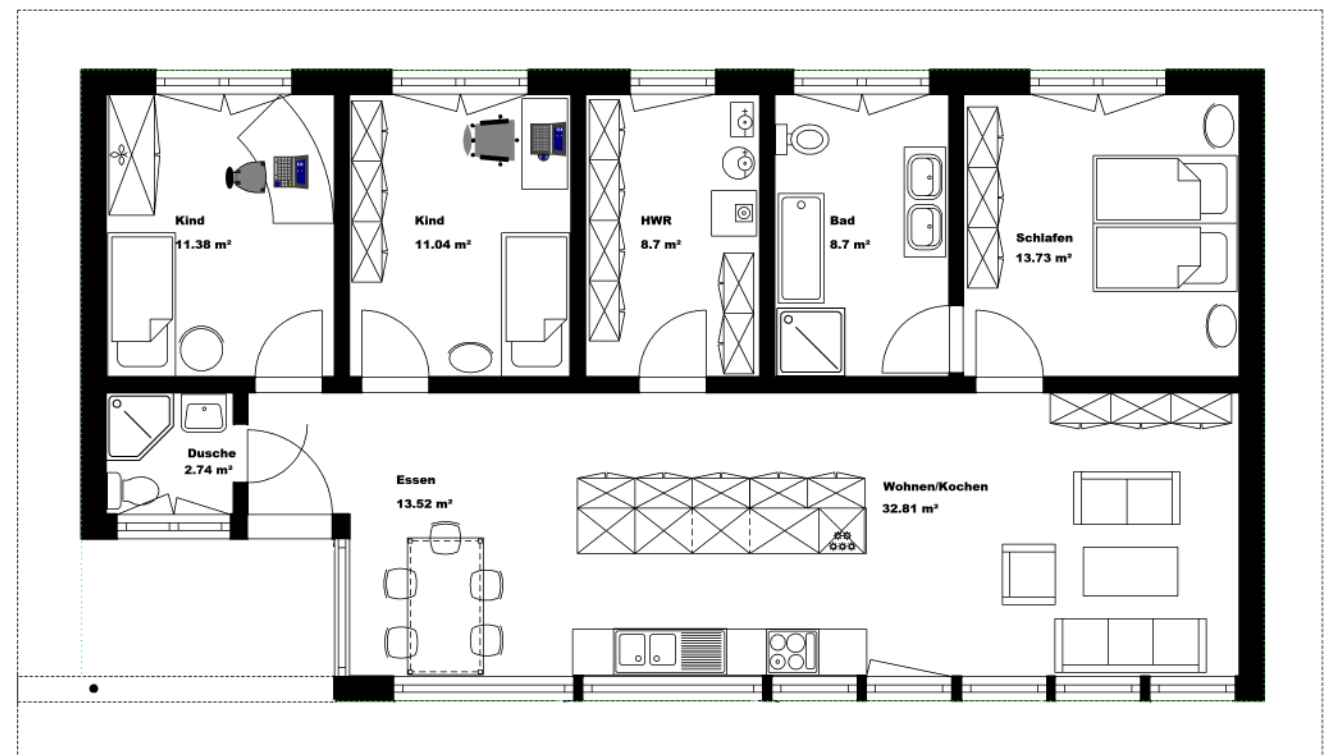
ERDGESCHOSS
